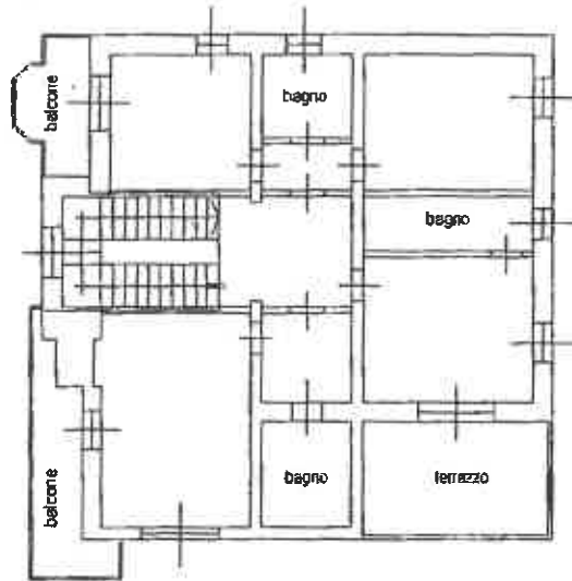
PIANTA PIANO PRIMO h. loc. = 3,90 m
