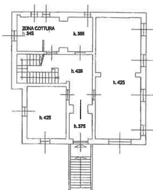
PIANTA PIANO TERRENO H. loc = 4,25 mt
